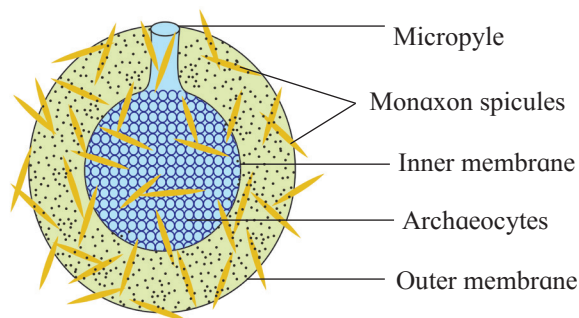
Fig. 2.1 : Gemmule
